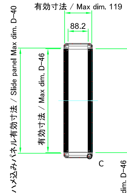
B-B ( 1 : 10 )
